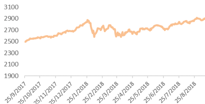
S&amp;P 500
